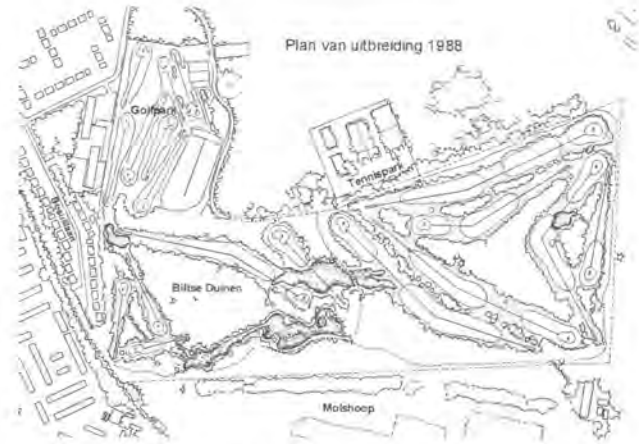
Het ontwerp uit 1988 voor de uitbreiding van het golfpark met een 9 holes golfbaan in de Biltse Duinen. (Bron: Golf Development International NV, Van Empelen Van Aalderen BV, Grontmij NV)
